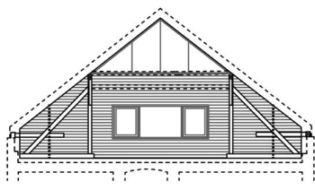
Ansicht Aussenwand Ost 1:200
